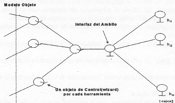
Figura N° 6. Esquema de objetos por ámbito.
