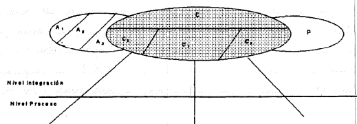
Figura Nº 4. Agente PAC raíz correspondiente al Nivel de Integración de la arquitectura PAC-OOCE
