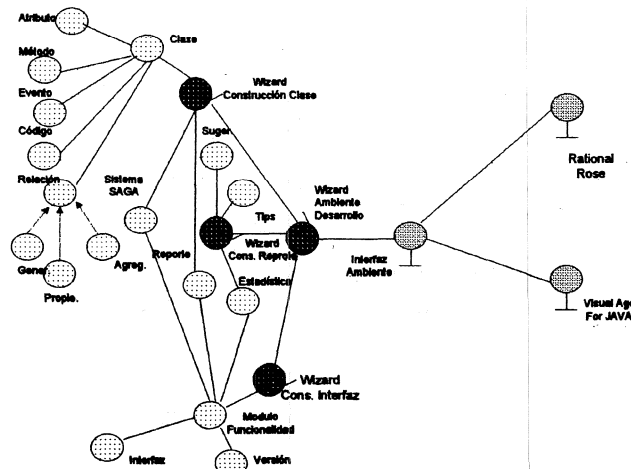
Figura N° 11. Esquema de Objetos del Ámbito Desarrollo de SAGAOOCE
