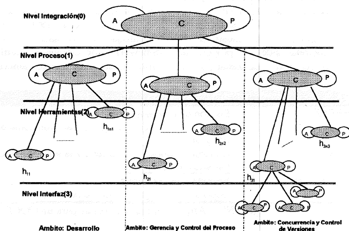
Figura Nº 3. Arquitectura PAC- OOCE
