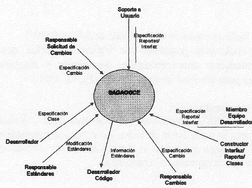
Figura N° 8. Modelo de Contexto del SAGAOOCE
