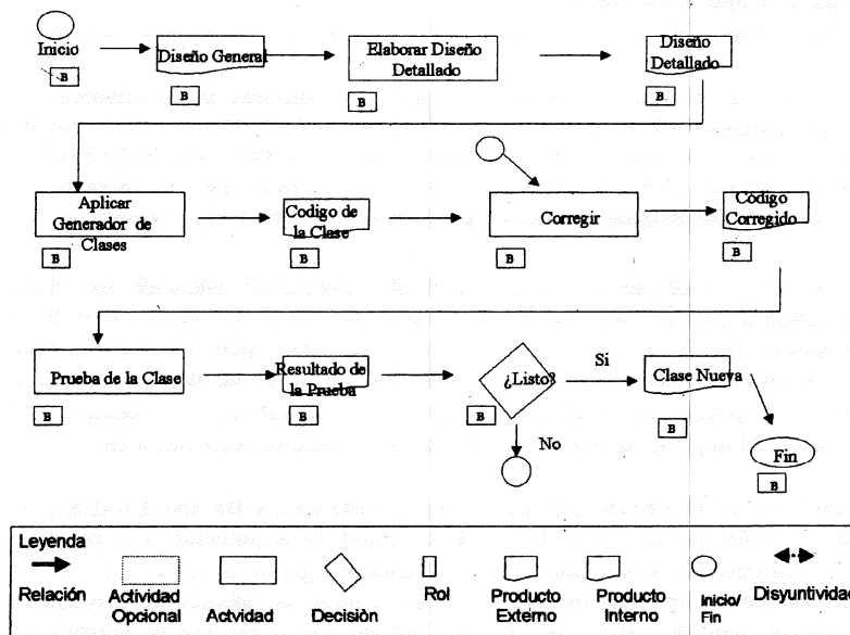
Figura N° 7. Especificación del Subproceso Construcción de Clases
